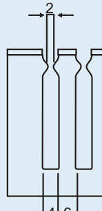
THIN SLOT
